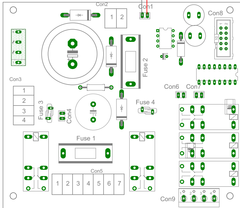
Output 24V DC
